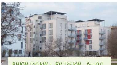
BHKW 140 kW el , PV 135 kW p , f p =0,0
