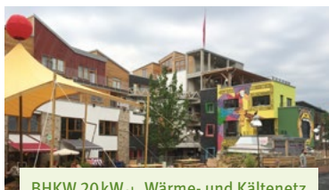
BHKW 20 kW el , Wärme- und Kältenetz
